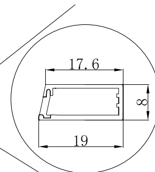
截面图
