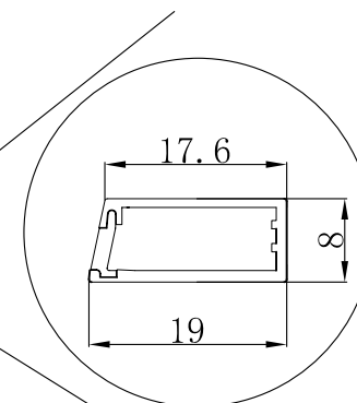
截面图
