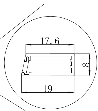
截面图
