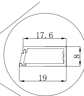
截面图
